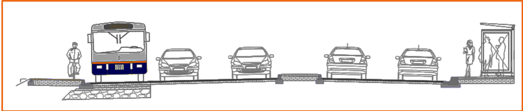
Coupe secteur Frênes-Dide
